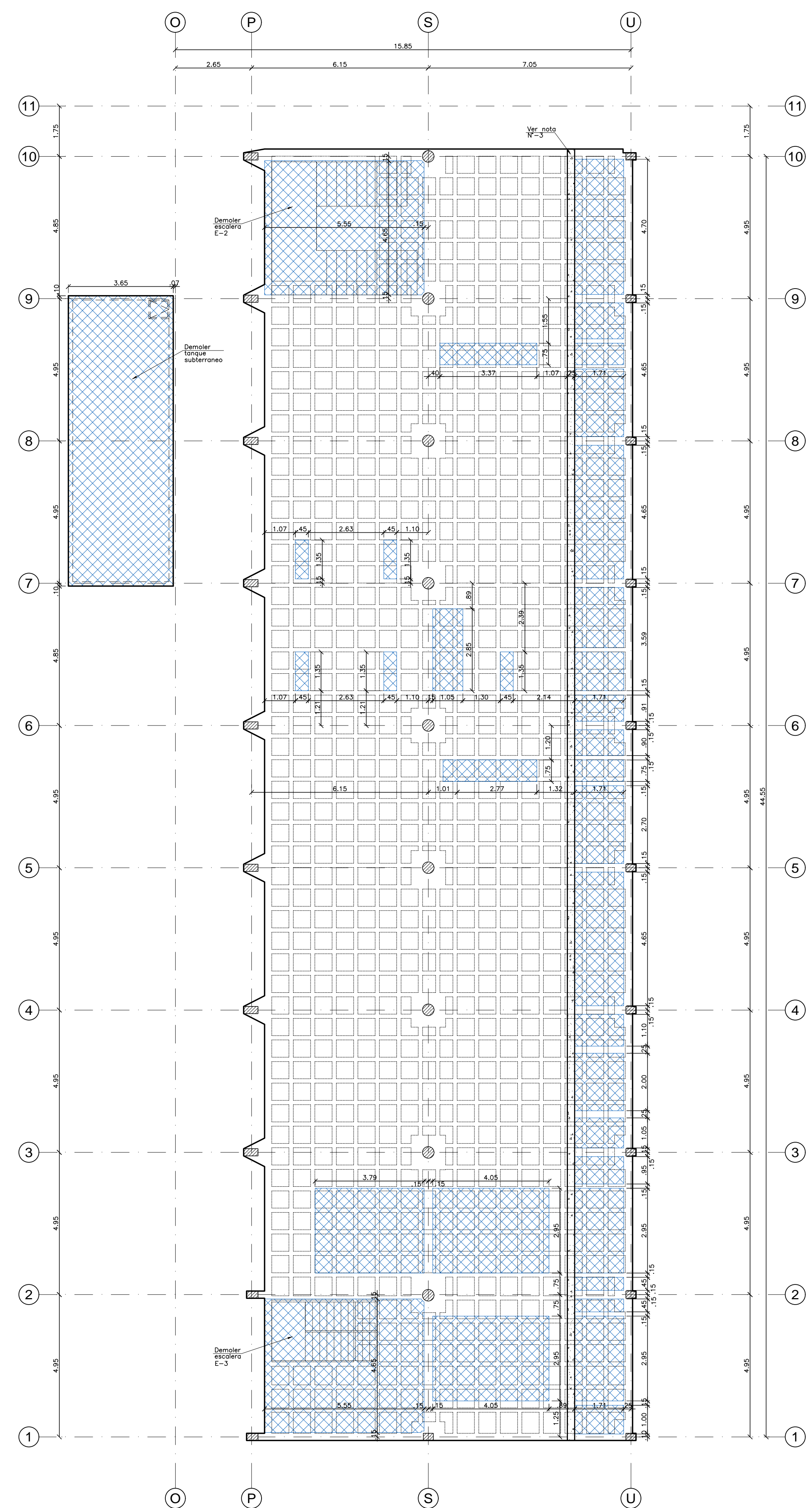
ESTRUCTURA 1 BLOQUE 2 - PLANTA PISO 1 NE+3.32 - DEMOLICIÓN ESCALA 1:100
